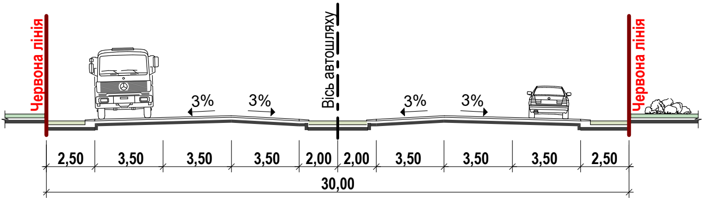
Поперечний профіль вулиці Демократична М 1:200
